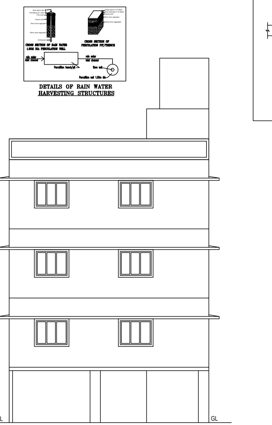
ELEVATION
